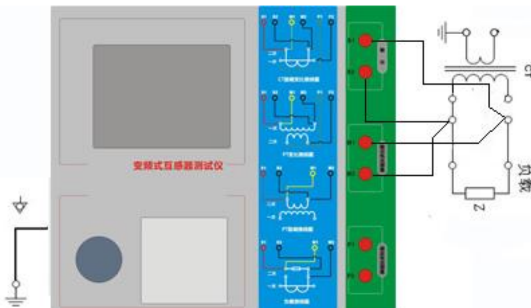
图 2.2 CT 二次负荷试验接线方式
