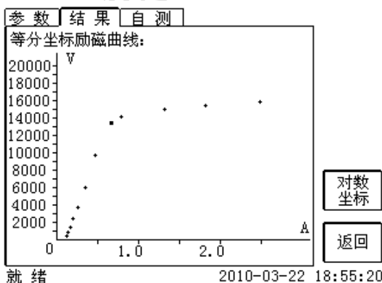
图 2.19 励磁曲线界面
