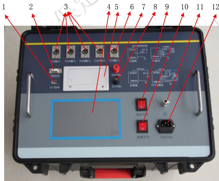
仪器面板 图 9
