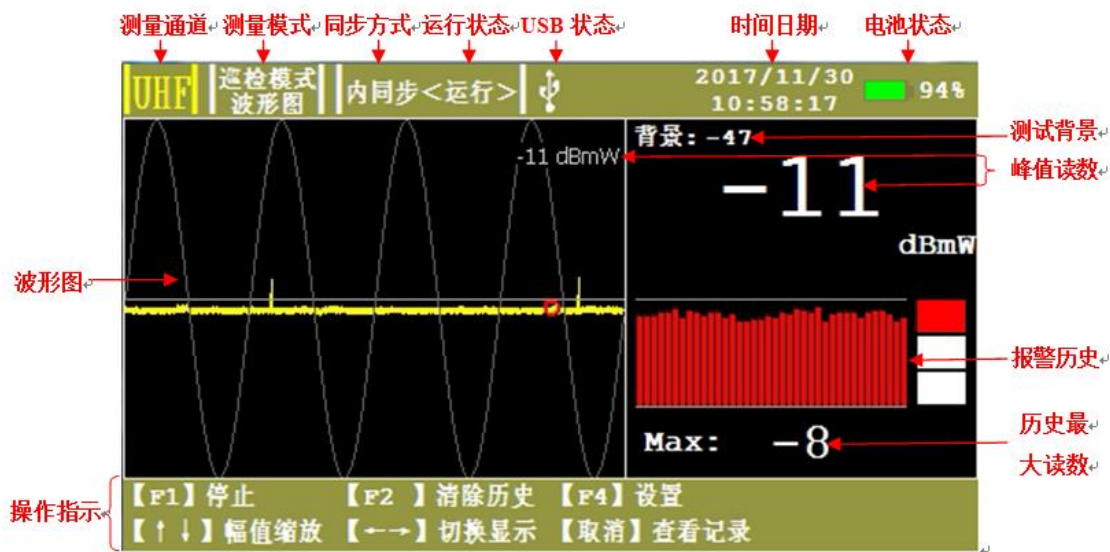
图1-12 UHF 波形图
