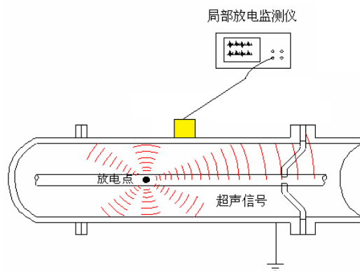
图1-2 GIS 局放超声检测原理图
